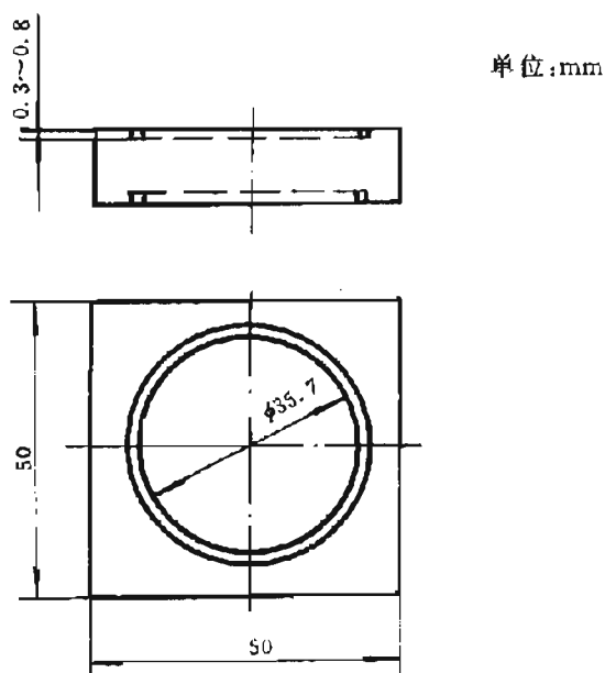
图 19 试件制作图
