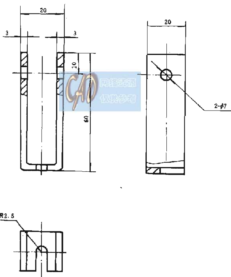
图 10 卡具 2 示意图
