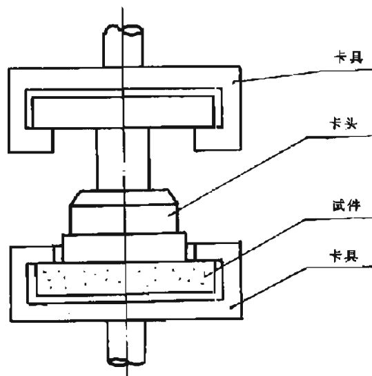
图 20 卡具夹持示意图
