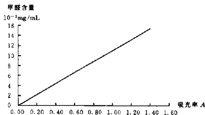
图 15 标准曲线
