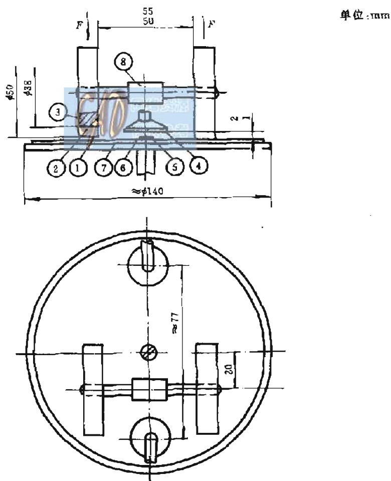
1—砂纸;2—橡胶;3—研磨轮;4—吸尘嘴;5—螺钉; 6—试件;7—试件夹;8—研磨轮提升装置
