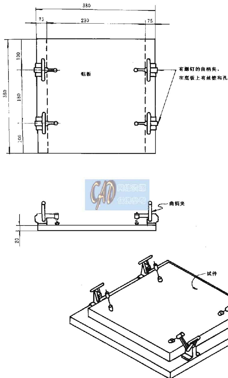
图 37 框式夹具
