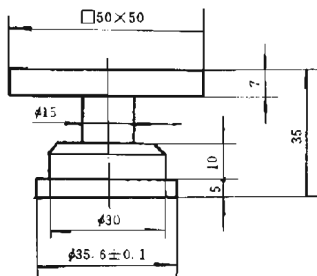
图 18 专用卡头
