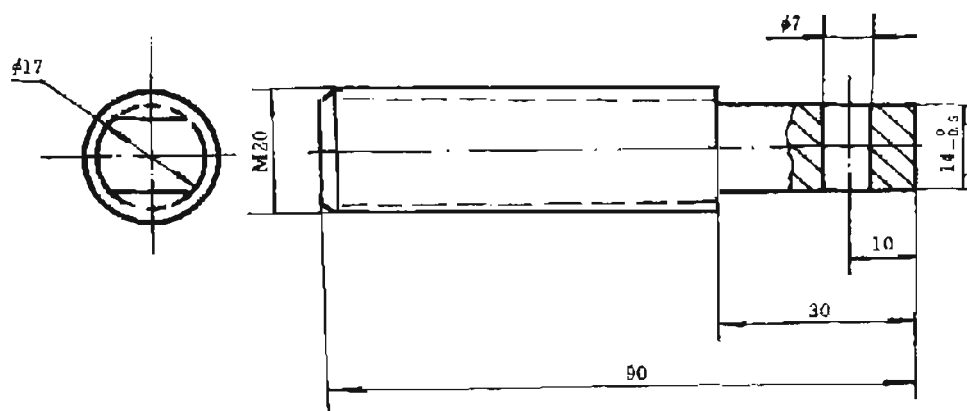
图 9 卡具 1 示意图
