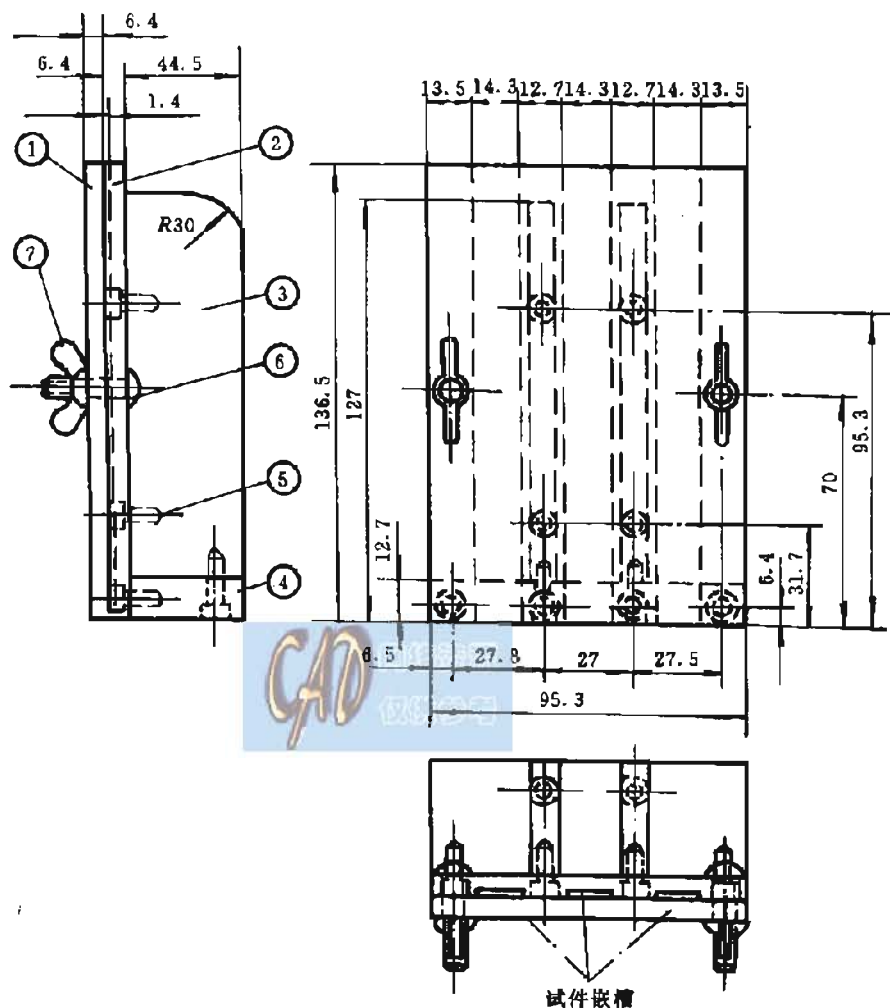
图 32 刚性夹具
