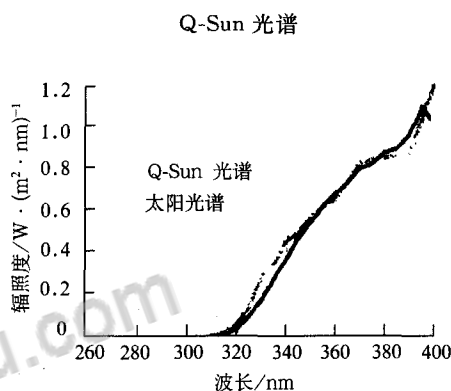
图1 Q-Sun光谱与太阳光谱
